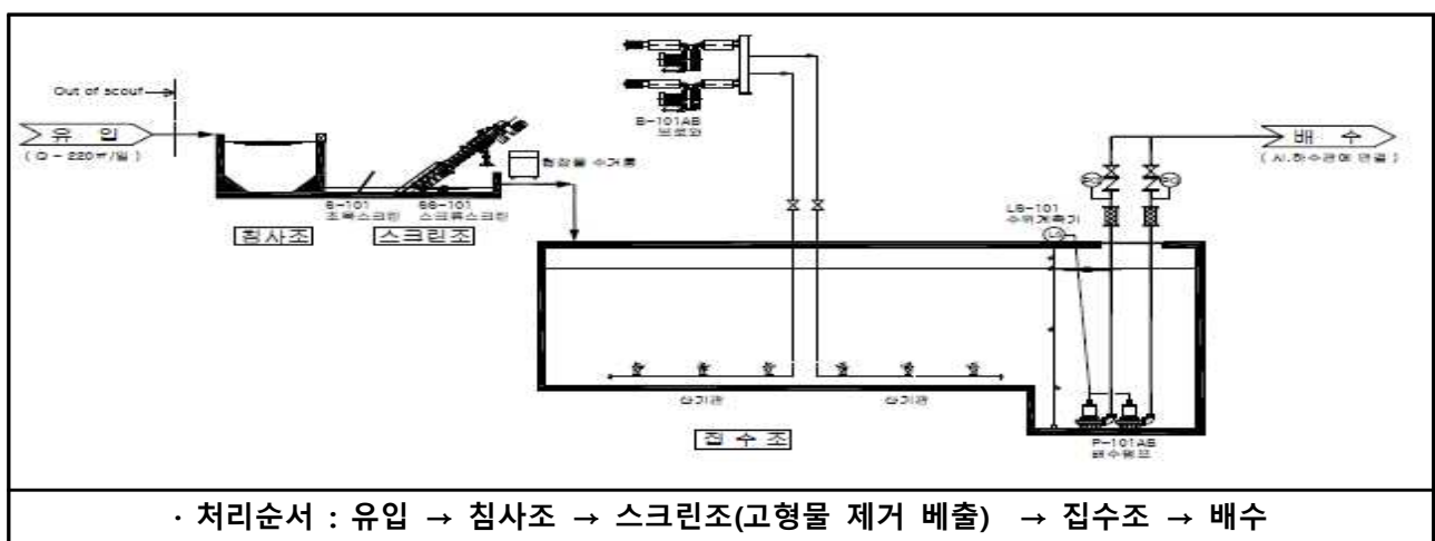
[표 2] 오수펌핑 처리 계통도
